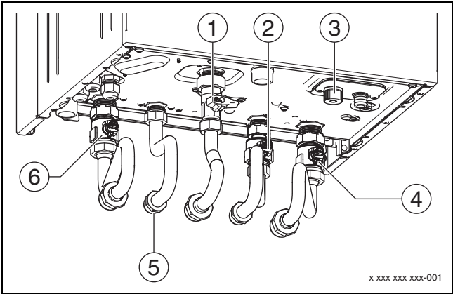
Fig. 11 Raccords côté gaz et eau xDOS GA 18
