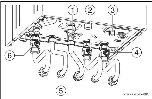
Fig. 10 Raccords côté gaz et eau xDOS GA 16
