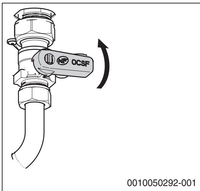
Fig. 5 Ouvrir le robinet de gaz xDOS GA 6/7/8/16/18
