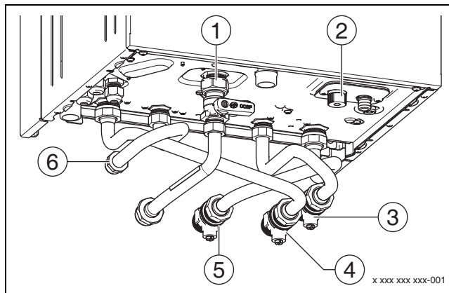
Fig. 7 Raccords côté gaz et eau xDOS GA 6
