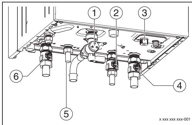
Fig. 6 Raccords côté gaz et eau xDOS GA 5/xDOS GA 15
