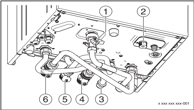
Fig. 8 Raccords côté gaz et eau xDOS GA 7
