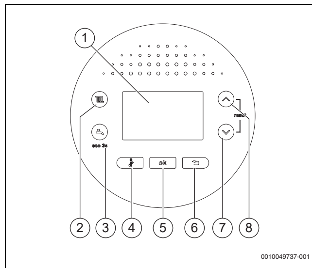
Fig. 3 Aperçu du tableau de commande
