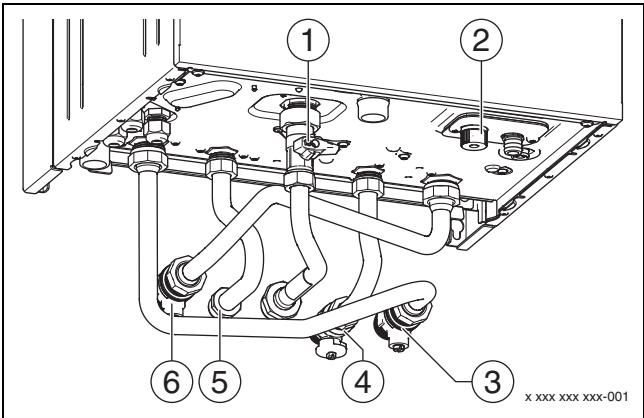
Fig. 9 Raccords côté gaz et eau xDOS GA 8
