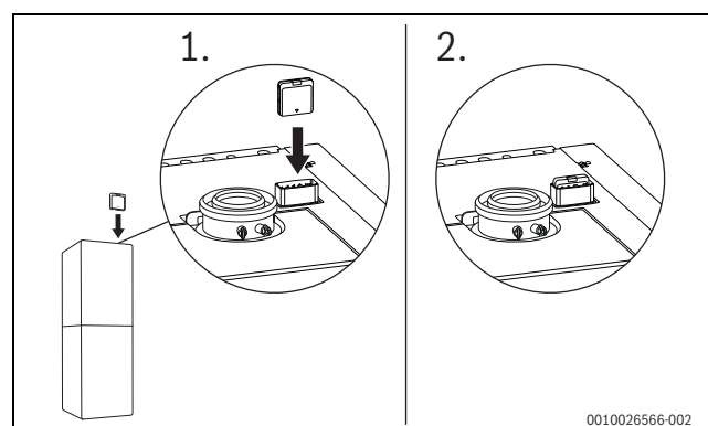
Fig. 2 Insérer le Control Key dans le support du Key
