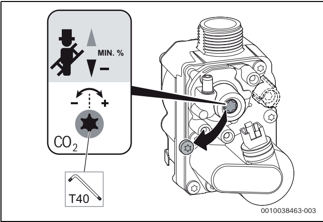
Fig. 91 Régler la teneur en CO 2 /O 2 sur la puissance thermique nominale minimale
