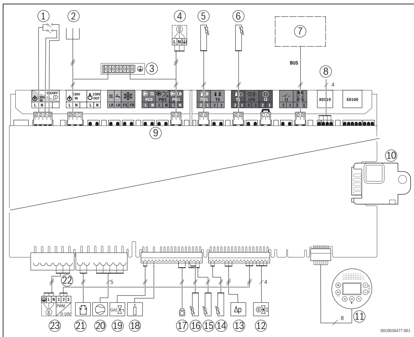
Fig. 139 Câblage électrique
