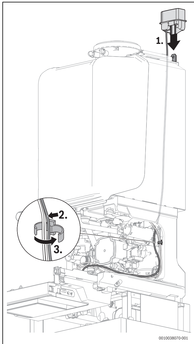
Fig. 51 Insérer le support de Key dans l'emplacement et fixer le câble dans le support de câbles
