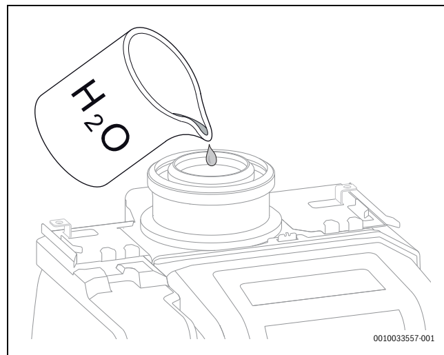
Fig. 57 Remplir le siphon des condensats avec de l'eau
