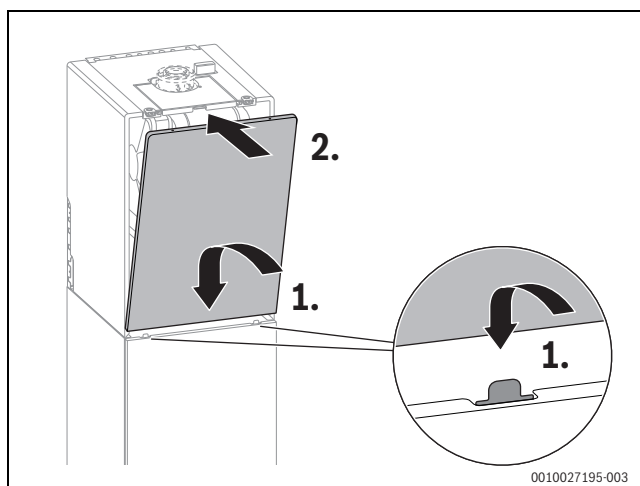
Fig. 76 Mettre en place le panneau avant de l'habillage
