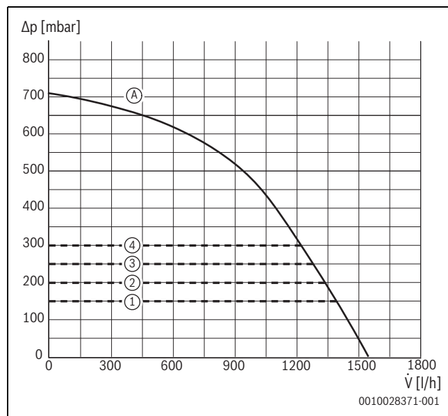
Fig. 140 Diagrammes de pompe et courbes caractéristiques de pompe (17/24 kW)
