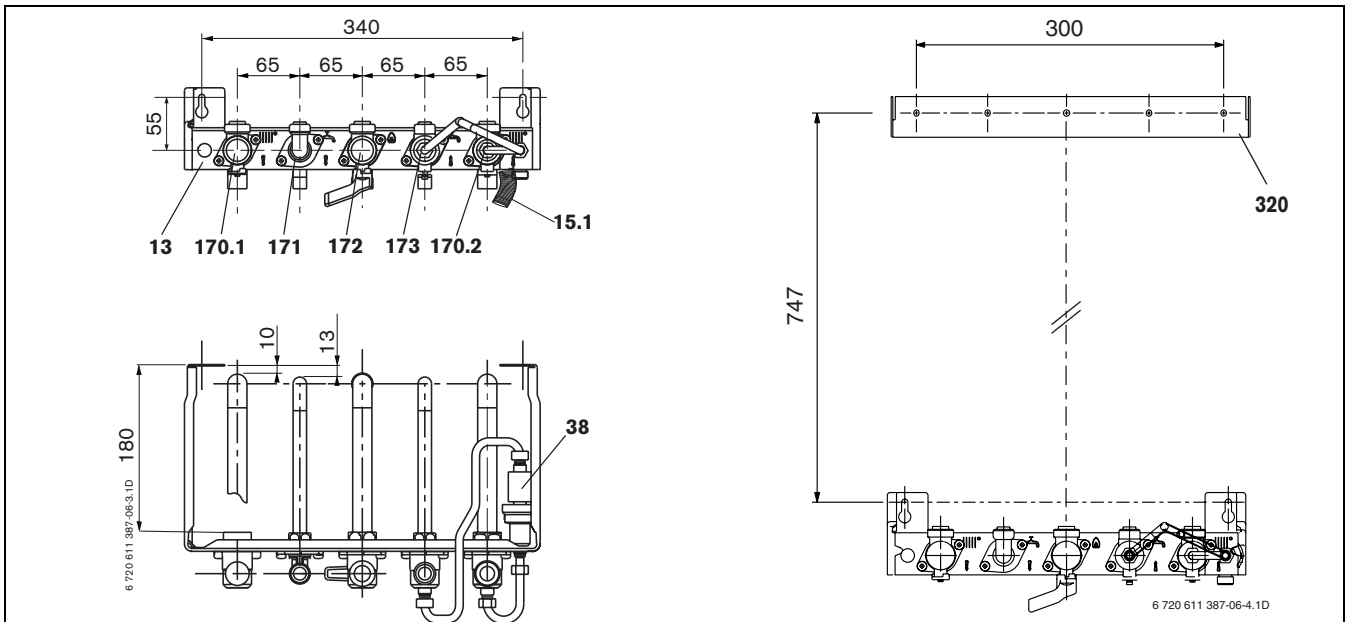
Fig. 3 Plaque de robinetterie avec barre d'accrochage GVAC (DOSGA5)
