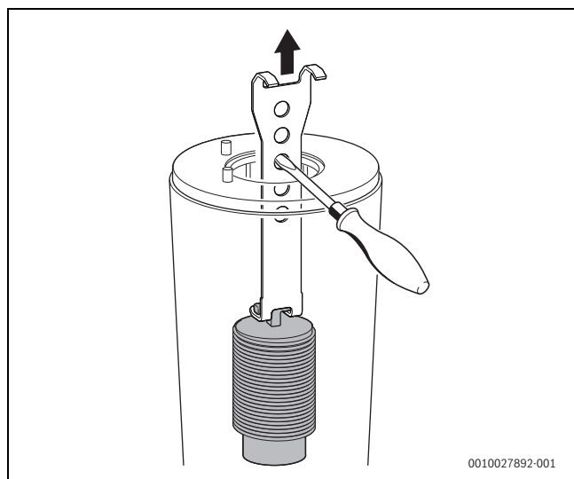
Fig. 50 Retirer le déflecteur inférieur
