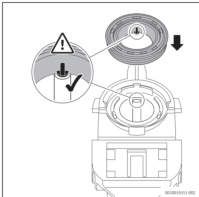
Fig. 59 Alignement du nouveau joint sur le siphon de condensats
