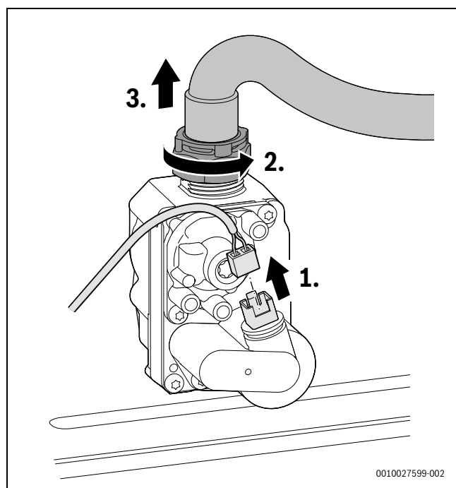
Fig. 64 Retrait du connecteur du bloc gaz et de l'écrou avec le tuyau du gaz
