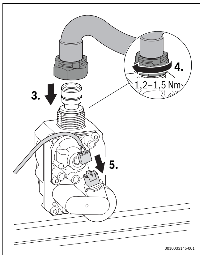
Fig. 71 Raccordement du tuyau du gaz et du connecteur – Respect du couple de serrage
