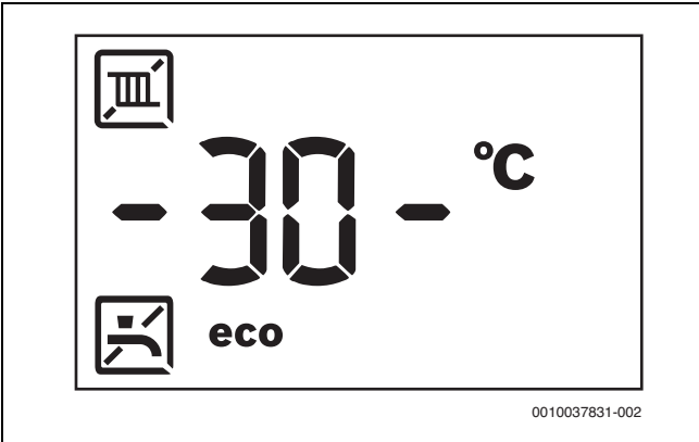
Fig. 35 La température de départ est affichée entourée de traits clignotants
