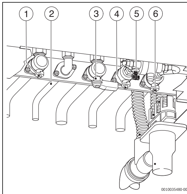
Fig. 28 Raccordements côté gaz et eau
