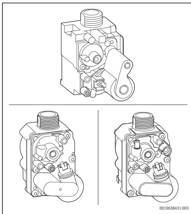
Fig. 36 En haut et en bas à gauche: vanne gaz fixe, en bas à droite: vanne gaz ajustable
