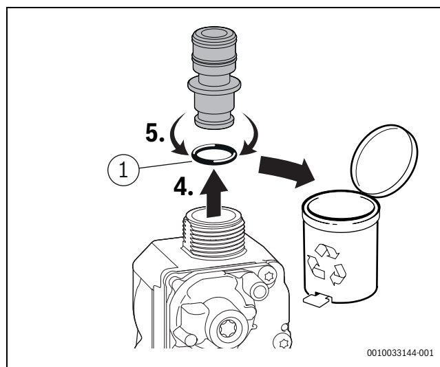
Fig. 65 Retrait de l'orifice
