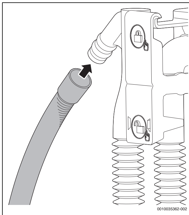
Fig. 24 Monter le tuyau des condensats sur le siphon de condensats.
