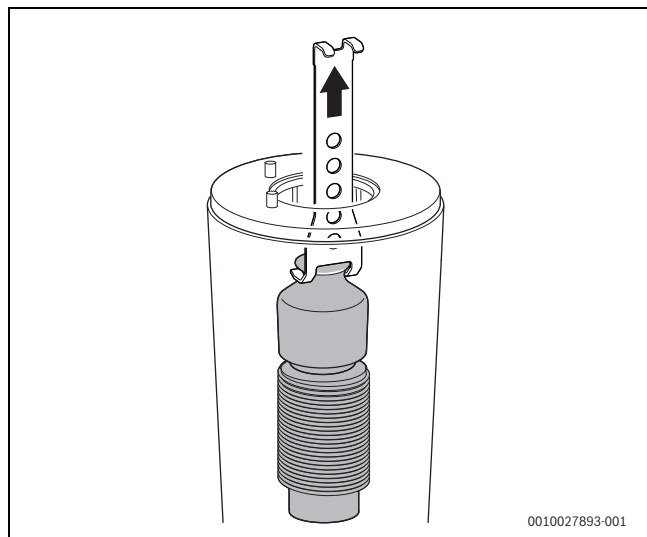
Fig. 49 Retirer le déflecteur supérieur
