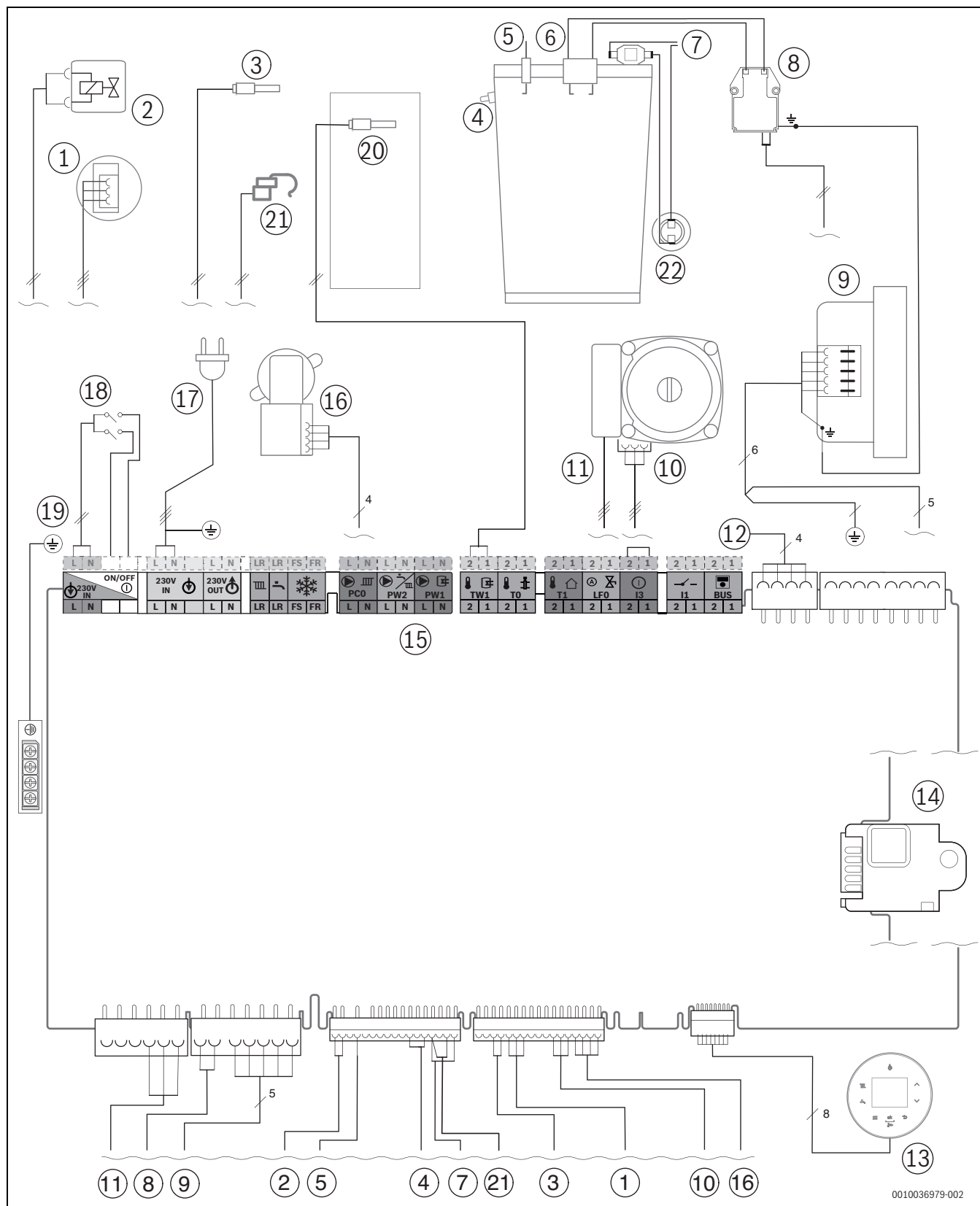
Fig. 77 Câblage électrique
