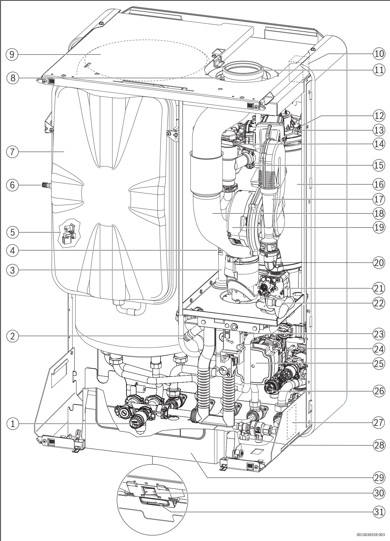
Fig. 4 Aperçu produit
