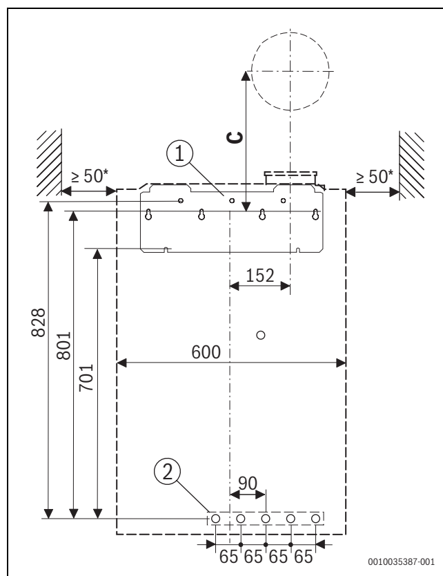
Fig. 3 Vue avant (mm)
