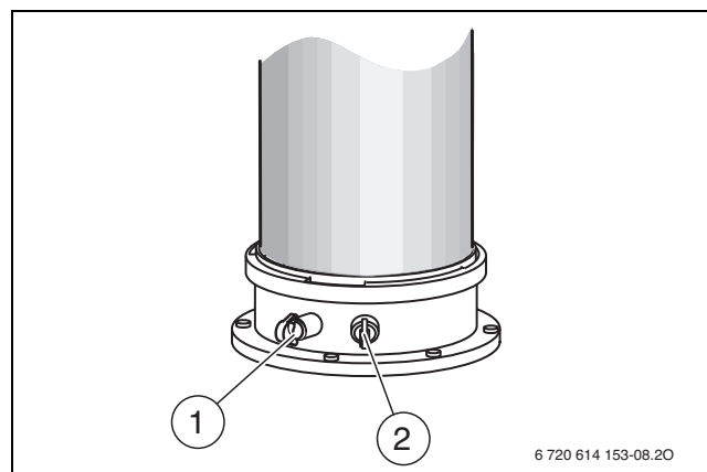
Fig. 42 Tubulure de mesure des fumées et de l'air de combustion
