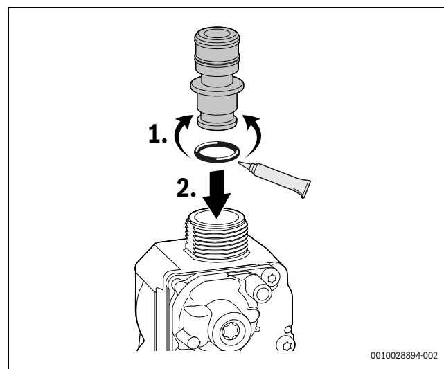
Fig. 70 Insertion l'orifice de réglage de gaz
