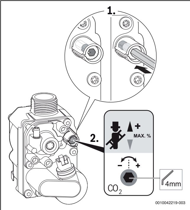
Fig. 40 CO 2 /O 2 -Régler la teneur en CO 2 /O 2 sur la puissance thermique nominale maximale, vanne gaz ajustable
