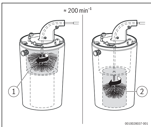
Fig. 53 Nettoyage du corps de chauffe (env. 200 tr/min, rotation à droite uniquement)
