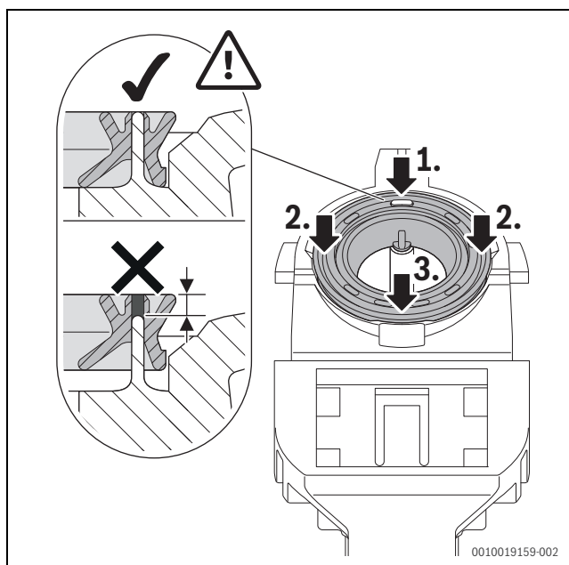
Fig. 60 Appui sur le joint
