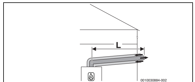
Fig. 7 Circuit d'air et de fumées concentrique horizontal selon C 13x par le mur extérieur
