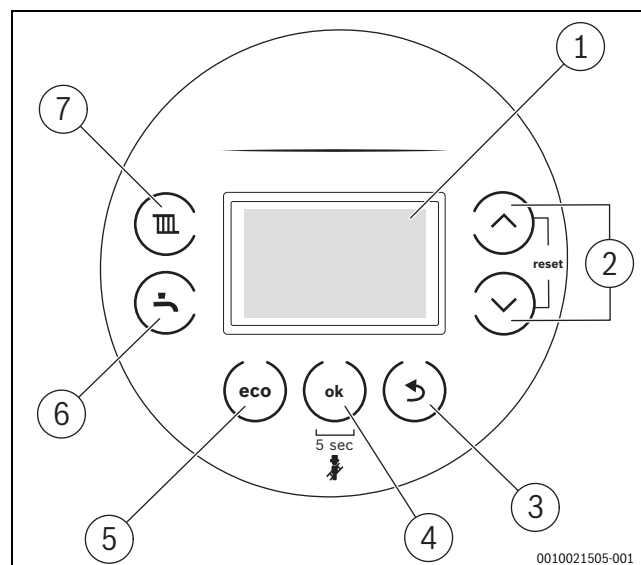
Fig. 34 Tableau de commande
