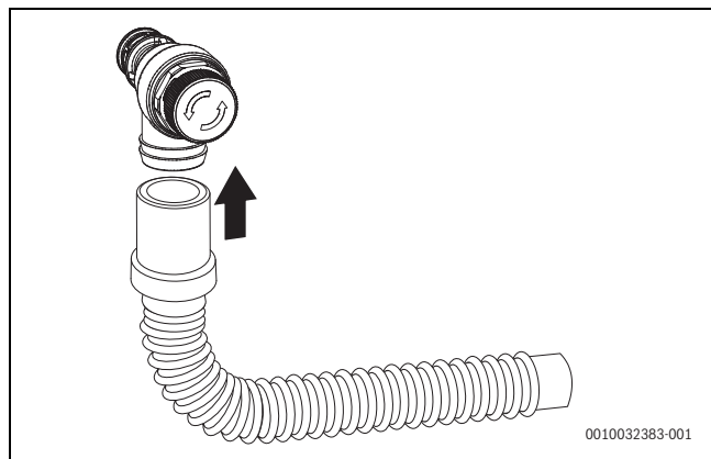
Fig. 22 Montage du tube sur la soupape de sécurité (chauffage)
