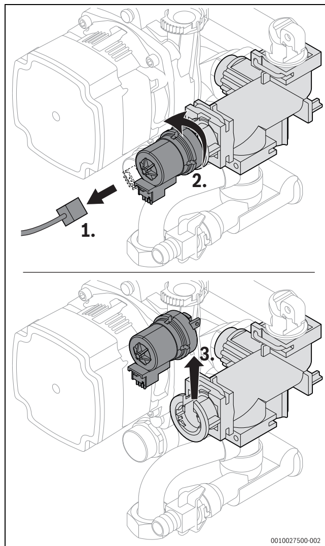
Fig. 72 Démonter le moteur au niveau de la vanne 3 voies (variante sans vis)
