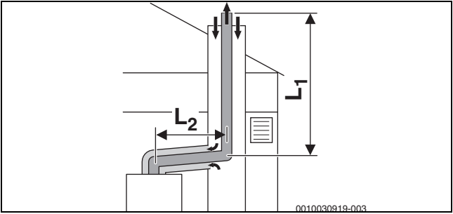
Fig. 9 Evacuation des fumées rigide selon C 93x dans le conduit et circuit d'air et de fumées concentrique dans le local d'installation
