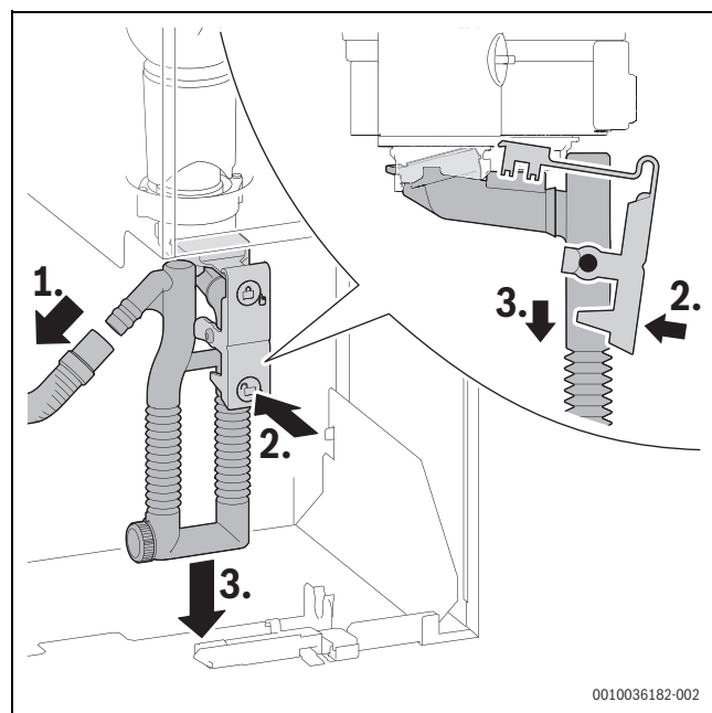
Fig. 56 Démontez le siphon des condensats
