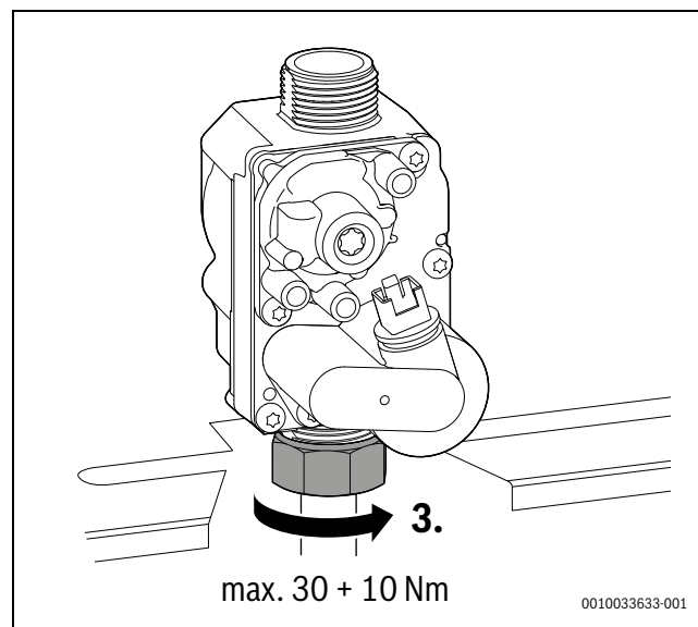
Fig. 69 Respect du couple de serrage
