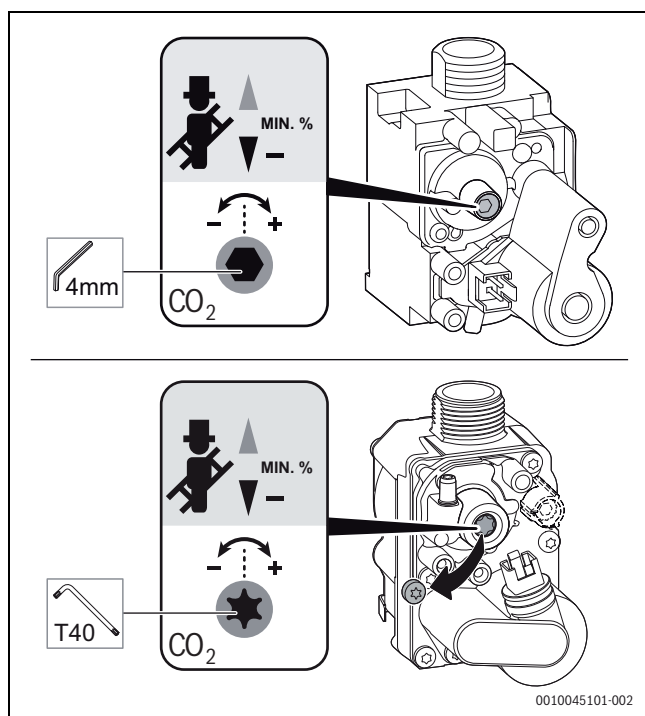
Fig. 41 Régler la teneur en \text{CO}_2/\text{O}_2 sur la puissance thermique nominale minimale
