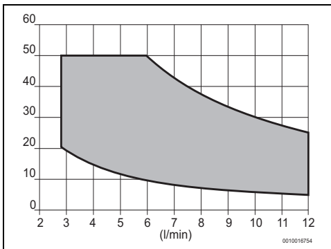
Fig. 32 Modèle 12 litres
