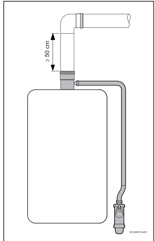
Fig. 17 Siphon des condensats (gaine technique horizontale)
