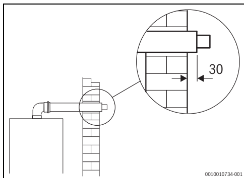
Fig. 25 Dimensions (en mm)
