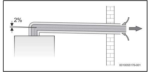
Fig. 23 Installation du type C13
