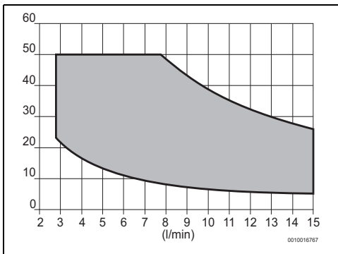
Fig. 32 Modèle 15 litres
