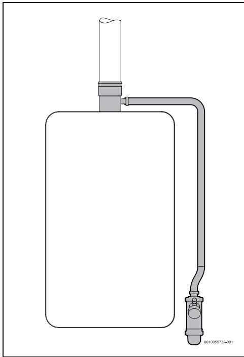
Fig. 16 Siphon des condensats (gaine technique verticale)
