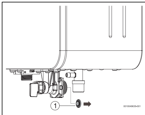
Fig. 29 Filtre à eau
