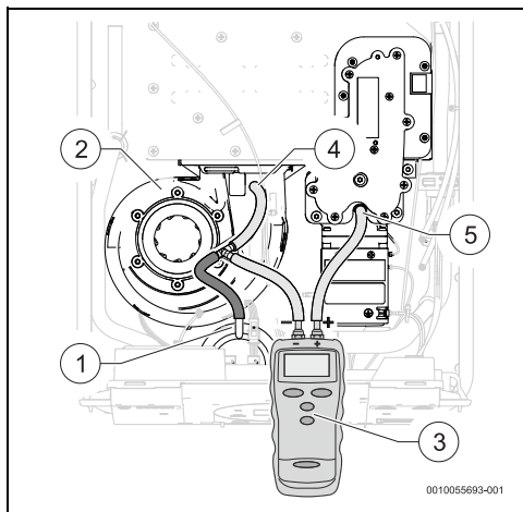
Fig. 28 Raccordement au ventilateur, capteur de pression et point de contrôle de pression
