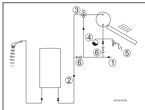
Fig. 18 Installation solaire
