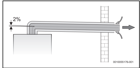
Fig. 23 Installation du type C13
