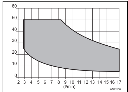
Fig. 34 Modèle 17 litres
