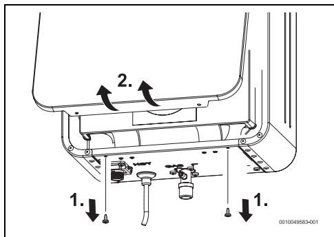
Fig. 28 Démontage de l'habillage avant
