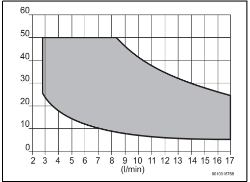
Fig. 33 Modèle 17 litres
