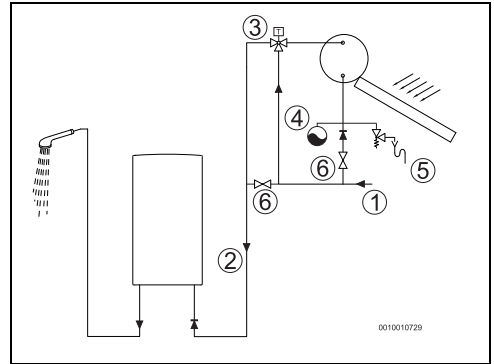
Fig. 18 Installation solaire
