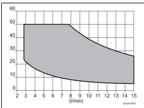
Fig. 33 Modèle 15 litres
