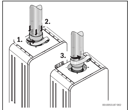
Fig. 24 Installation du type B23
