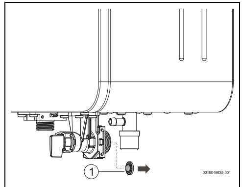
Fig. 30 Filtre à eau
