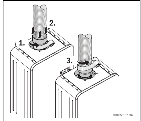
Fig. 24 Installation du type B23
