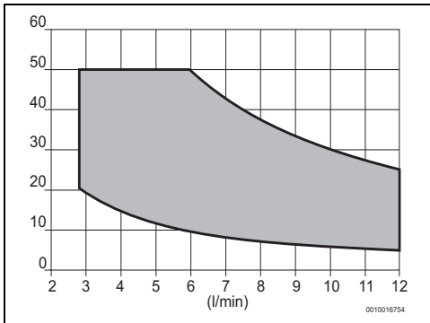
Fig. 31 Modèle 12 litres
