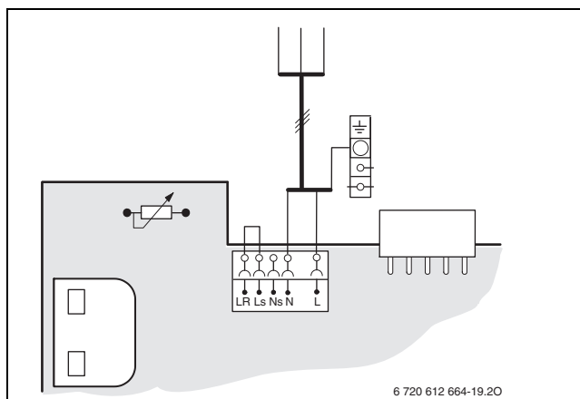
Fig. 49 Bornier d'alimentation secteur ST10
