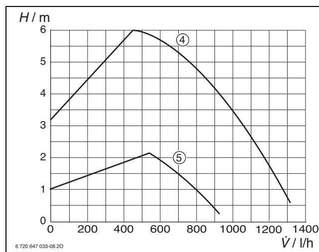
Fig. 63 Pression proportionnelle
