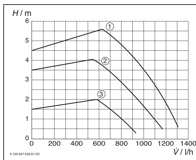
Fig. 62 Pression constante
