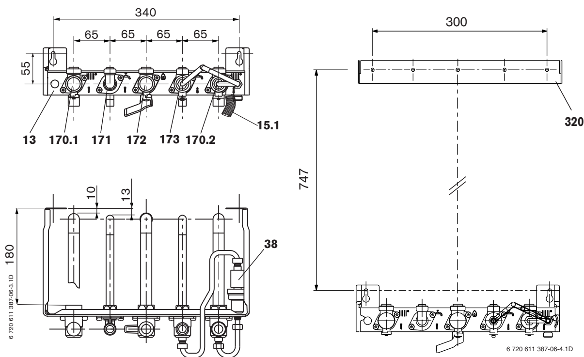
Fig. 5 Plaque de robinetterie
